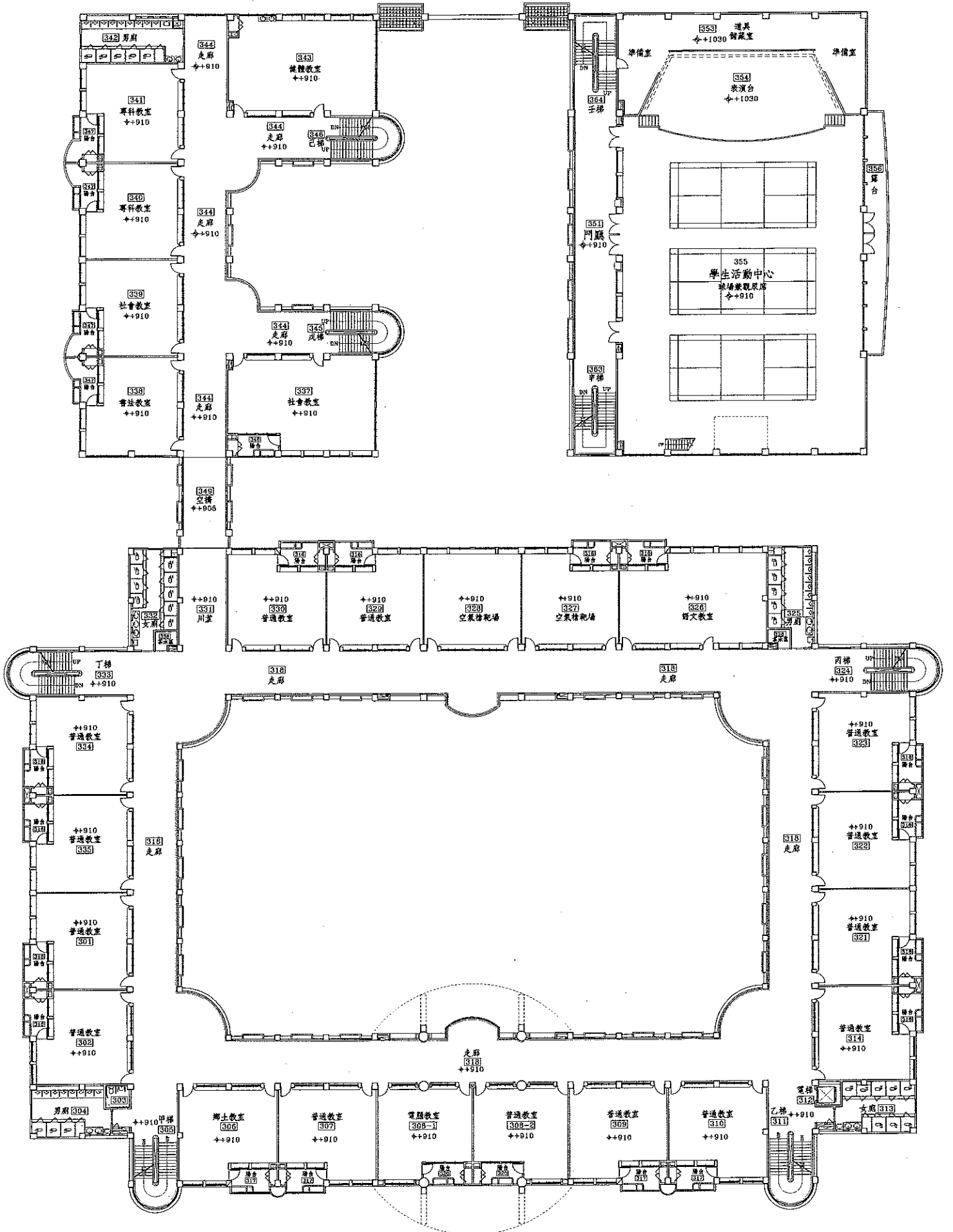
參層平面圖 S:1/300
