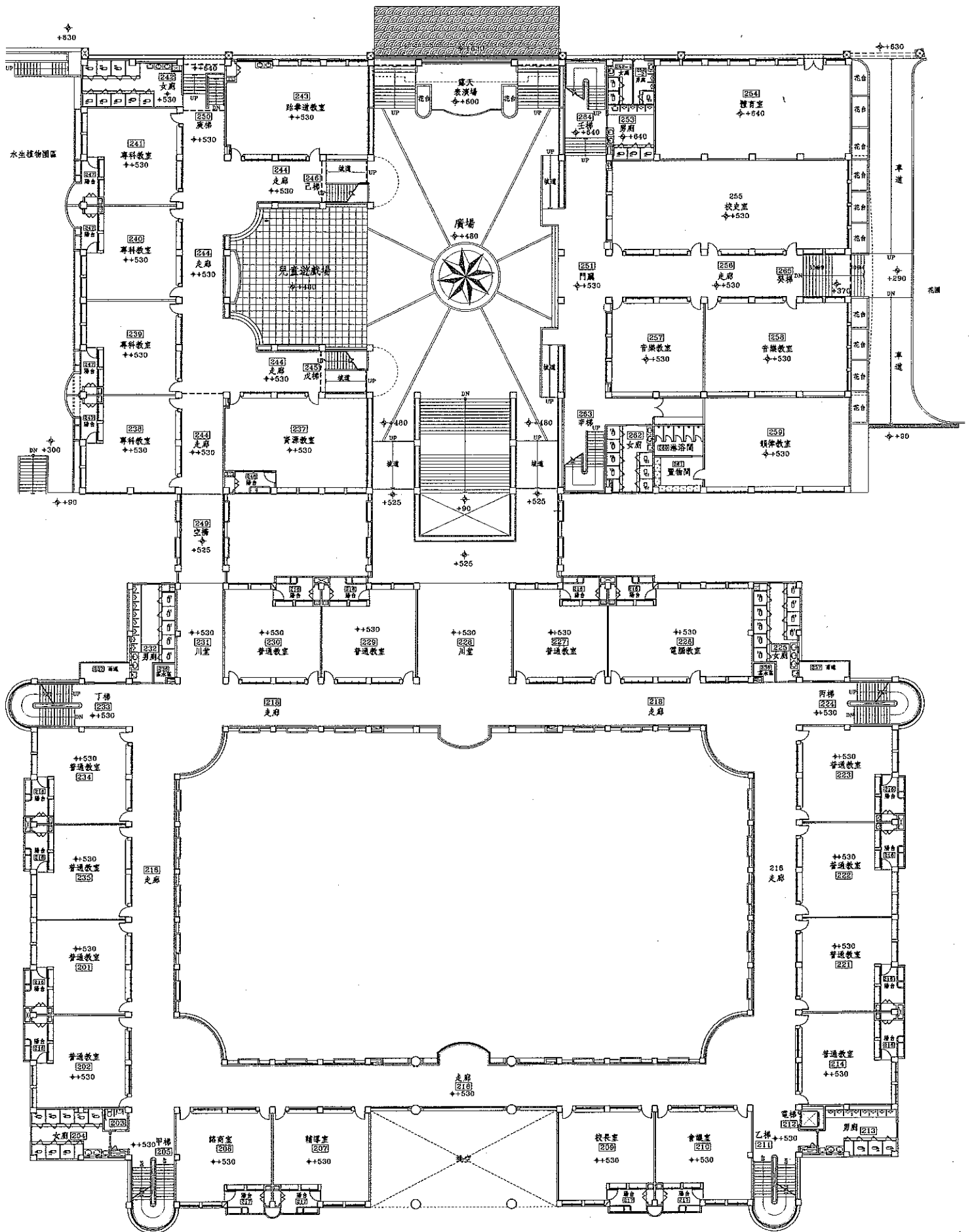
貳層平面圖 S:1/300
